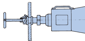
Einsatz durch Zapflochklappe Mounting with clap
