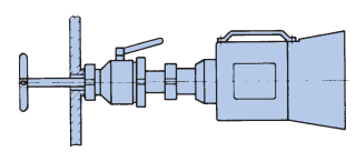
Einsatz durch Kugelhahn Mounting with ball valve
